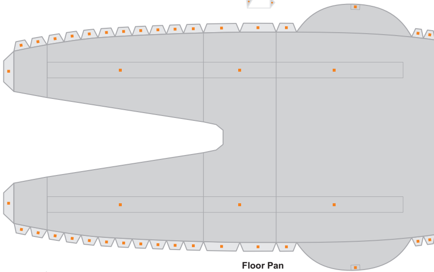
Floor Pan Piso del Carro
