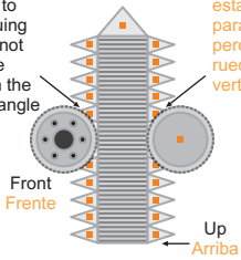
Blower (Upper) Pulley Polea de Supercargador (Superior)
